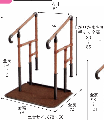
土台サイズ78×56
