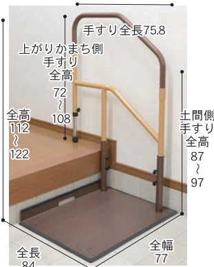
土台サイズ77×58
